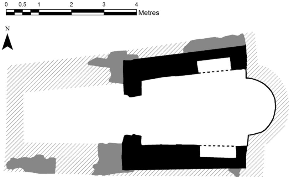
Εικ. 10 Η Παναγία Θεοσκέπαστη: Κάτοψη της υπάρχουσας κατάστασης (μαύρο), με ορατά τα ερείπια τειχών (γκρι) και διαγραμμισμένους τους πιθανούς, πρωιμότερους τειχούς. Το πάχος του υπάρχοντος νότιου τειχους είναι άγνωστο. (Sam Turner & Alex Turner).
