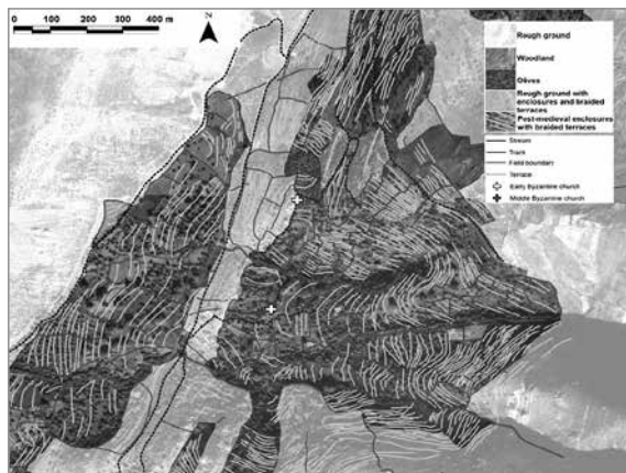
Εικ. 2 Ιστορικός Χαρακτηρισμός Τοπίου και ανάλυση ΓΣΠ στην περιοχή των Αριών στη Νάξο (περιέχει δεδομένα από IKONOS © 2006, Space Imaging LLC. All rights reserved).
